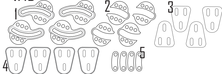
1. Demi-disque / Half disk 2. Entretoise / Crosspiece 3. Tôle PAD / Steel plate PAD 4. PAD / PAD 5. Languette / Strip
