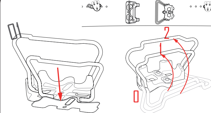
1. Braquet de montée / Ascent bracket 2. Support de câble / Heel riser holder 3. Tôle de protection / Protection steel plate 4. Câles / Steel thread
