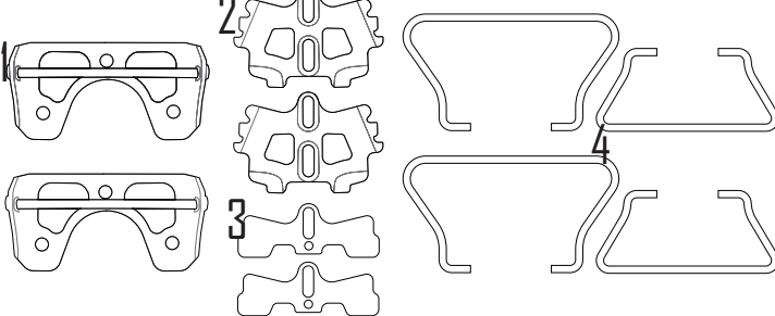
1. Braquet de montée / Ascent bracket 2. Support de câble / Heel riser holder 3. Tôle de protection / Protection steel plate 4. Câles / Steel thread
